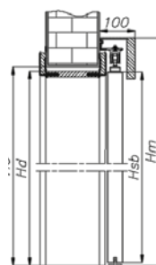
drzwi przesuwne - system naścienny bez zabudowy
