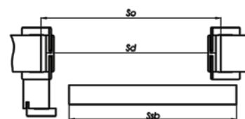
drzwi przesuwne - system naścienny z zabudową tunelową ZN
