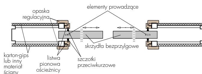
dwudzielne / przekrój poziomy
