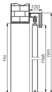
drzwi przesuwne - system naścienny bez zabudowy
