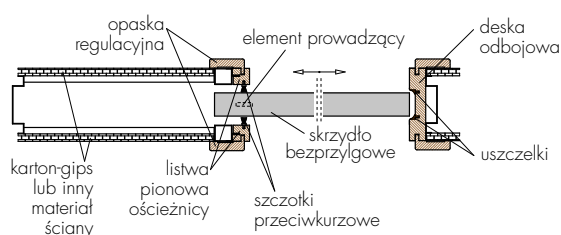
jednodzielne / przekrój poziomy
