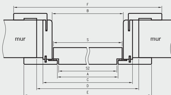
Przekrój poziomy ORO
