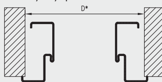
przekrój poprzeczny alternatywny sposób montażu
