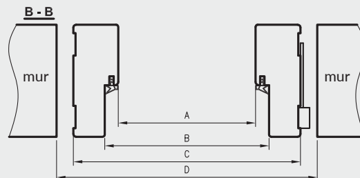
Przekrój poziomy
