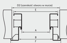
Przekrój poprzeczny przy montażu na zaprawę murarską
