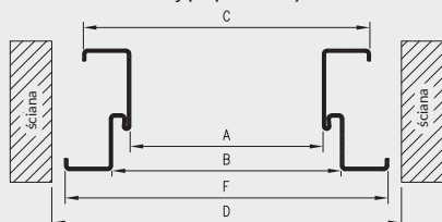
Przekrój poprzeczny
