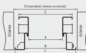
Przekrój poprzeczny przy montażu na wełnę mineralną
