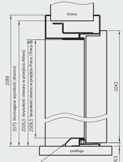
przekrój ościeżnicy stalowej regulowanej
