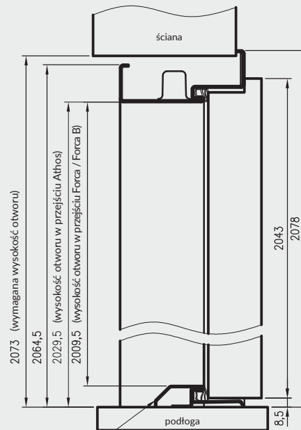
przekrój pionowy
