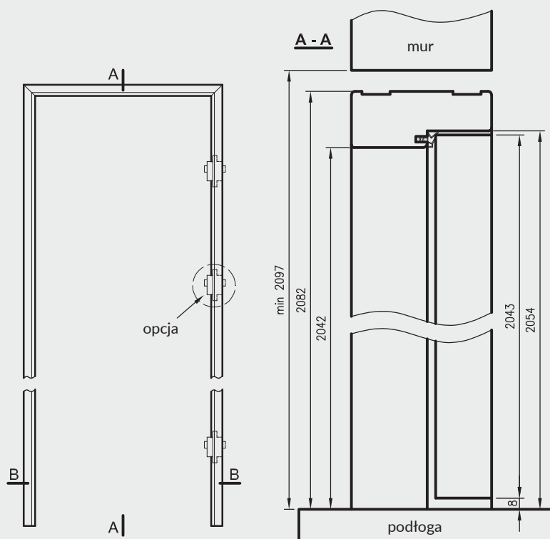
Przekrój pionowy drzwi bezprzylgowych OPB
