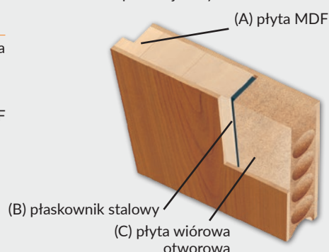
przekrój skrzydła ENTER natura
