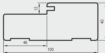
Przekrój poziomy
