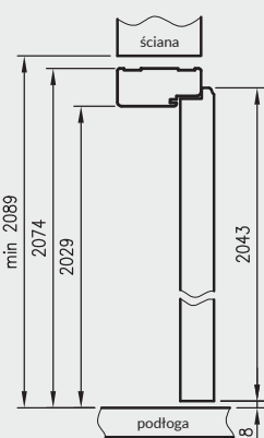
Przekrój pionowy drzwi przylgowych
