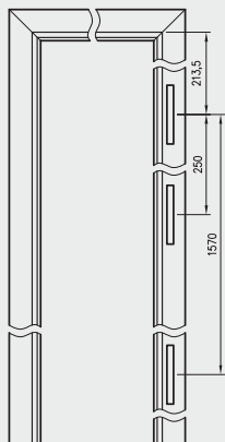
ościeznica metalowa pod zawiasy VX 7939
