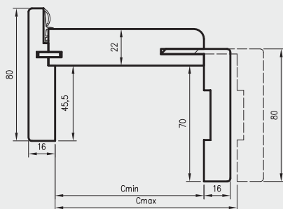
Przekrój pionowy ORO
