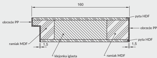
PRZĘKRÓJ RAMIĄKA PIONOWEGO
