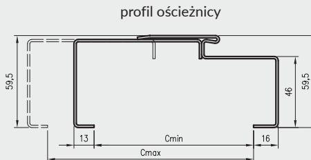
profil ościeżnicy
