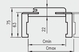
Przekrój OR/ORC z ką. T63
