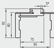
Przekrój ORB 075
