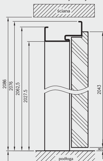
przekrój poprzeczny alternatywny sposób montażu
