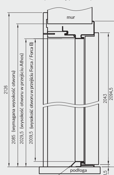
przekrój pionowy
