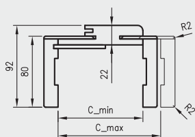
Przekrój ORB 075
