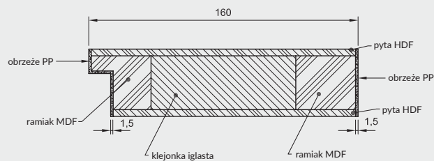
PRZEKRÓJ RAMIĄKA PIONOWEGO
