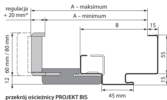
przekrój ościeznicy PROJEKT BIS
