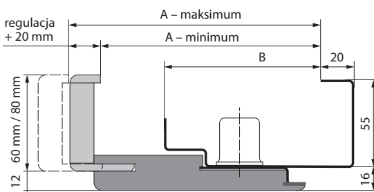
przekrój ościeznicy PROJEKT Premium
