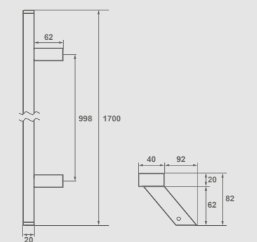
Amsterdam Skos 170 cm
