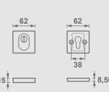
Mars Flex Click Rozeta
