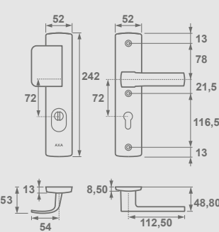
Apollo Flex Premium Klamko-pochwyty, rozstaw 72 mm
