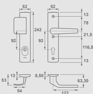
Arrow Flex Premium Klamko-pochwyty, rozstaw 92 mm
