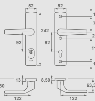
Arrow Flex Premium Klamko-klamka, rozstaw 92 mm
