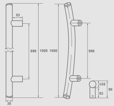
Montreal Gięta 150 cm
