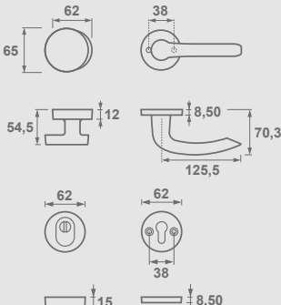
Diana Flex Premium Klamko-pochwyty
