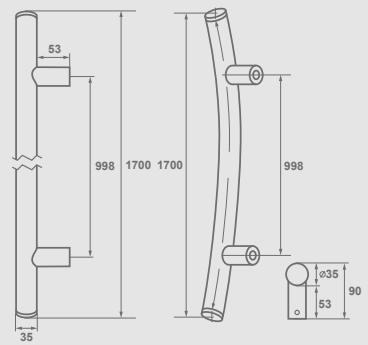
Montreal Gięta 170 cm
