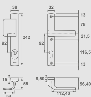
Solid Flex Premium Klamko-pochwyty, rozstaw 92 mm
