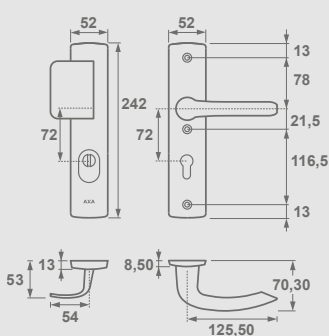
Jupiter Flex Premium Klamko-pochwyty, rozstaw 72 mm
