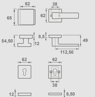
Mars Click Klamko-pochwyty
