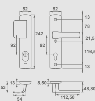
Apollo Flex Premium Klamko-pochwyty, rozstaw 92 mm
