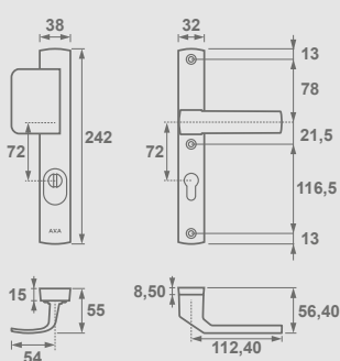
Solid Flex Premium Klamko-pochwyty, rozstaw 72 mm
