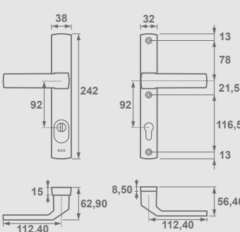
Solid Flex Premium Klamko-klamka, rozstaw 92 mm
