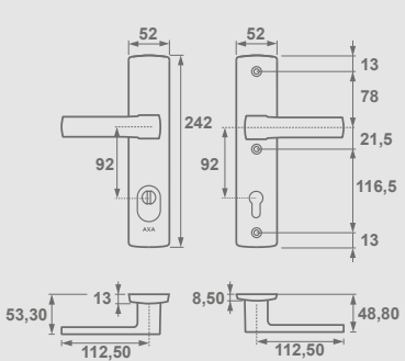
Apollo Flex Premium Klamko-klamka, rozstaw 92 mm
