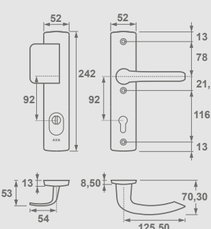
Jupiter Flex Premium Klamko-pochwyty, rozstaw 92 mm
