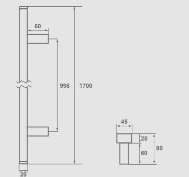
Amsterdam Prosta 170 cm
