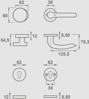
Diana Premium Klamko-pochwyty
