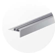
Profil Incizo / podprofil aluminiowy Incizo do schodów QSVINCP(-) / NEVINCPBASE1 2000 x 45 x 8 mm / 2000 x 33 x 17 mm
