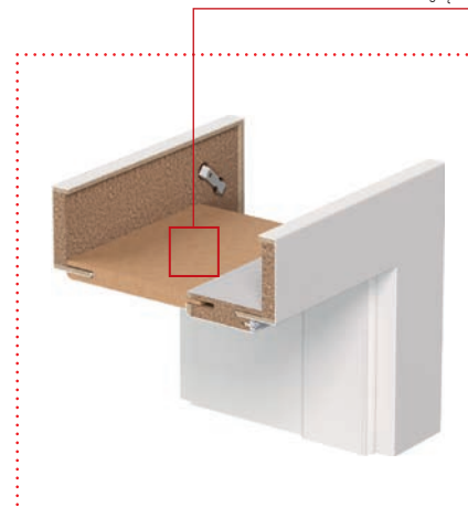
PRZĘKÓJ OŚCIEŻNICY Z PANELEM REGULUJĄCYM
