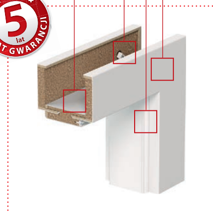
PRZĘKÓJ OŚCIEŻNICY PODSTAWOWEJ
