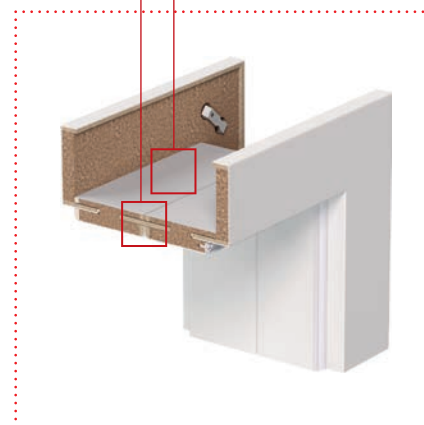
PRZĘKÓJ OŚCIEŻNICY ŁĄCZONEJ
