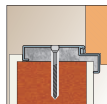
Montaż na dyble.
