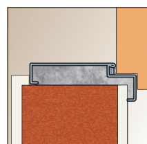
Montaż bez dodatkowych elementów kotwiących.
