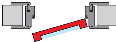
SPOSÓB MONTOWANIA SZYBY MATOWEJ (SKRZYDŁO PRAWIE – CZĘŚĆ MATOWA OD STRONY OBSERWATORA)
