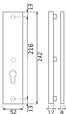
sztyld - widok z przodu i boku
