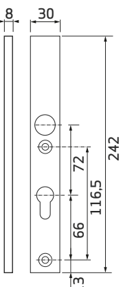
sztyld - widok z boku i przodu
