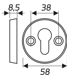
rozeta - widok z boku i przodu
