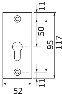
rozeta - widok z p. i boku
