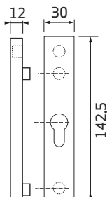
rozeta długa - widok z boku i p.
