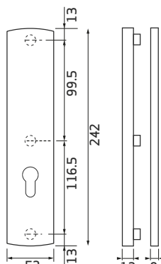
sztyld - widok z przodu i boku
