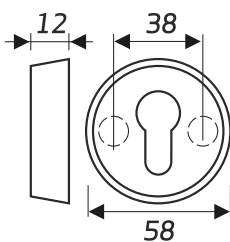
rozeta - widok z boku i przodu
