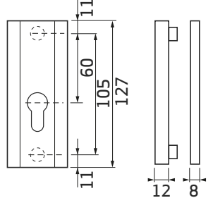
rozeta długa - widok z p. i boku
