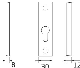
rozeta - widok z p. i boku
