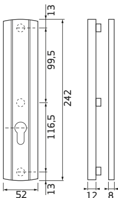
sztyld - widok z przodu i boku
