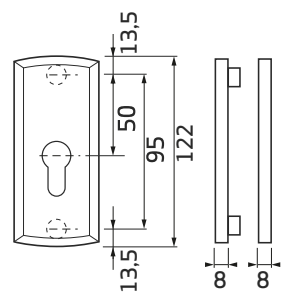
rozeta - widok z przodu i boku
