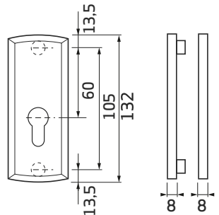
rozeta długa - widok z p. i boku
