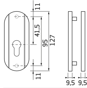
rozeta - widok z p. i boku
