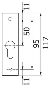
rozeta - widok z przodu
