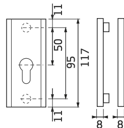
rozeta - widok z przodu i boku
