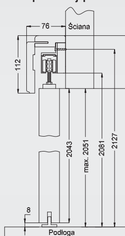
NS - przekrój pionowy
