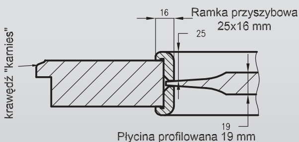
Konstrukcja skrzydeł Cell
