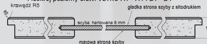
Przekrój poziomy drzwi VETRO A1 - A4 i B1 - B4
