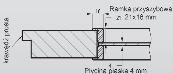
Konstrukcja skrzydeł Cell TOP
