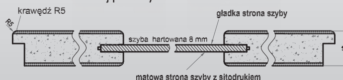
Przekrój poziomy drzwi VETRO A5 i B5
