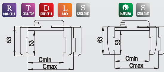
Przekrój ościeznicy regulowanej
