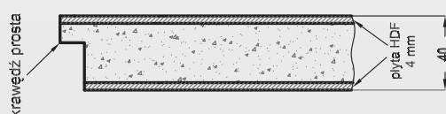
Drzwi Przeciwpożarowe (przekrój poziomy)
