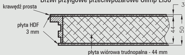
Drzwi przylgowe przeciwpożarowe Olimp EI30
