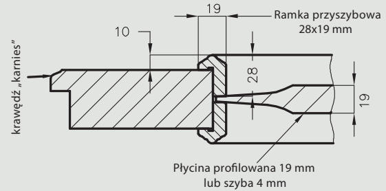
Konstrukcja skrzydeł przylgowych Natura
