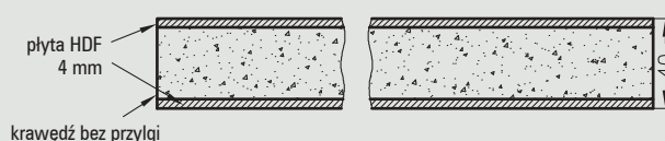
Drzwi bezprzylgowe rozwierne Finea TOP
