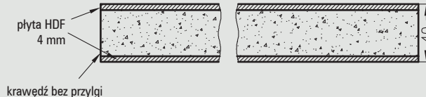
Drzwi przylgowe przeciwpożarowe Olimp EI60
