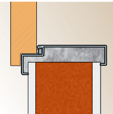
Montaż bez dodatkowych elementów kotwiących
