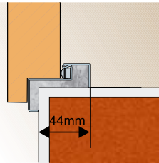
Ościeżnica kątowa mała
