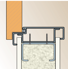
Ościeżnica kątowa duża montaż na ścianie kartonowo-gipsowej
