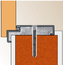
Ościeżnica kątowa duża montaż na dyble
