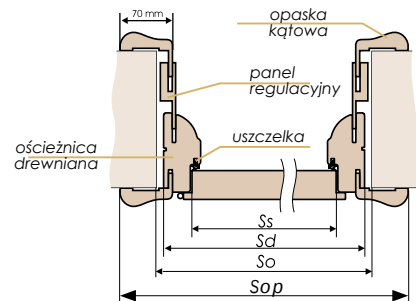
drzwi z ościeżnicą Regulowaną Model RETRO
