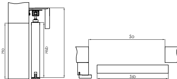
drzwi przesuwne – system naścienny bez zabudowy
