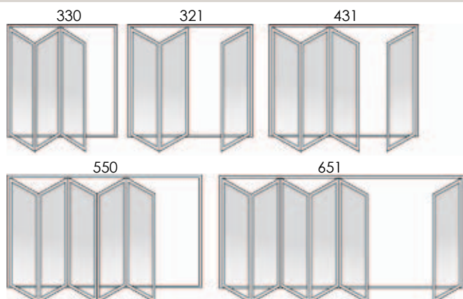
Przykładowe patio składane
