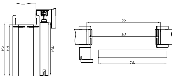
drzwi przesuwne – system naścienny z zabudową tunelową ZN OK6
