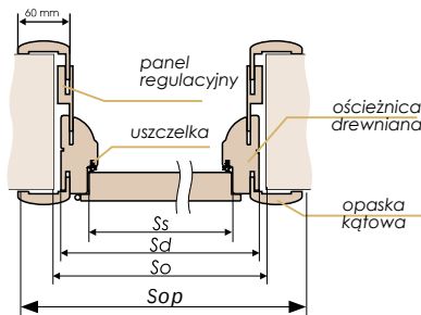
drzwi z ościeżnicą Regulowaną Model 2000
